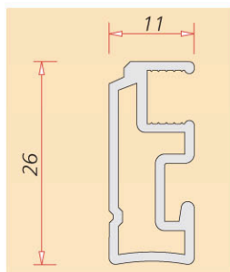
Dimensions du profil
