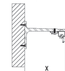
Fixation de face pour saillie de 75 à 250 mm
