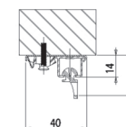
Fixation plafond
